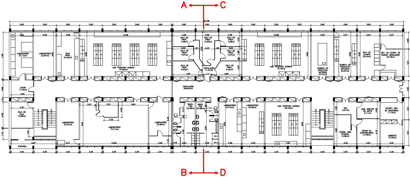
1 PLANTA BAIXA 1º PAVIMENTO ESCALA: S/ESC ÁREA DE CONSTRUÇÃO: 1.107,07m 2
